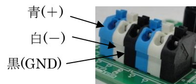
[端子部]
