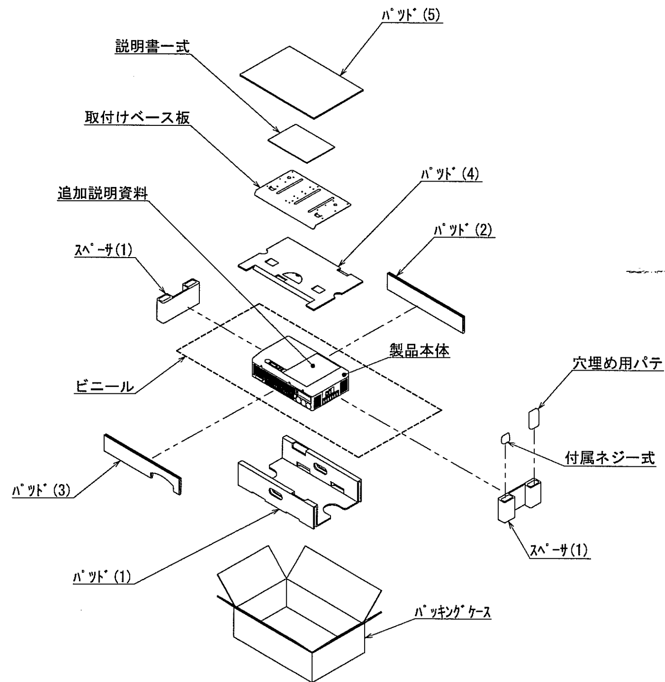
梱包内容説明図 (S=Free)
